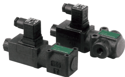
電磁操作ストップバルブ(HSOシリーズ)
