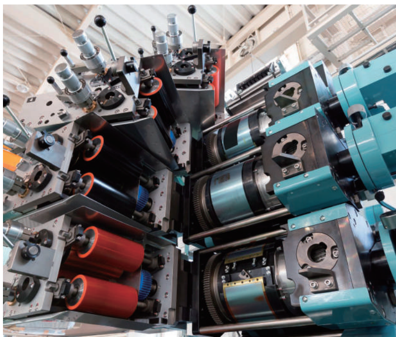
自社ブランド製品の曲面印刷機
